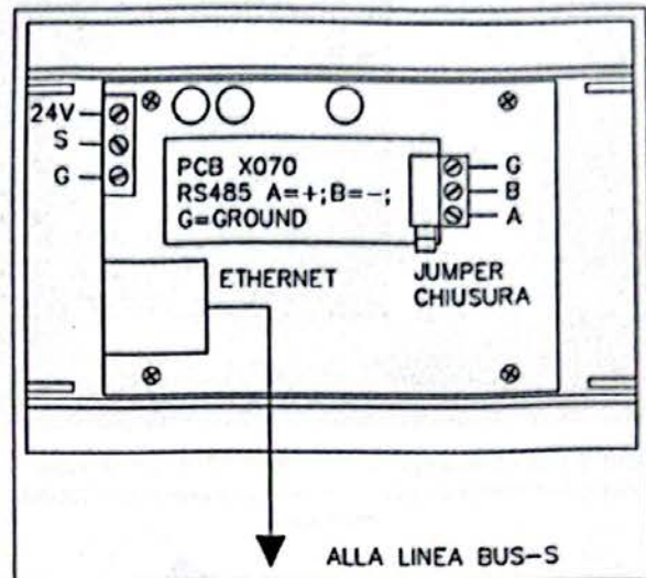
Connexion Tcp-ip/carte supplémentaire
