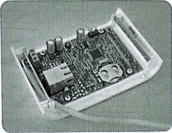
Introduire deux supports à droite et à gauche du panneau
