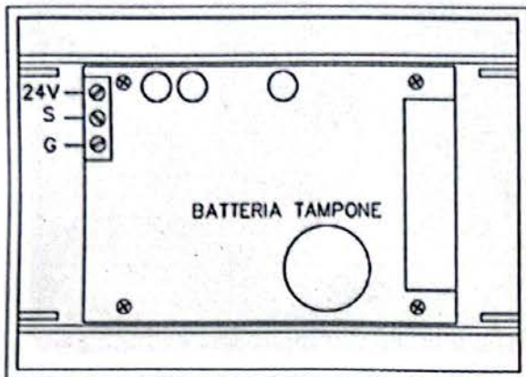
Panneau à distance : vue de derrière
