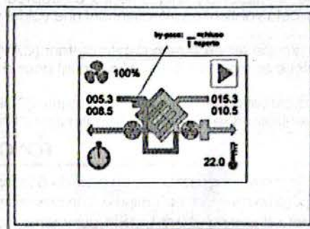
Groupe AVEC by-pass
