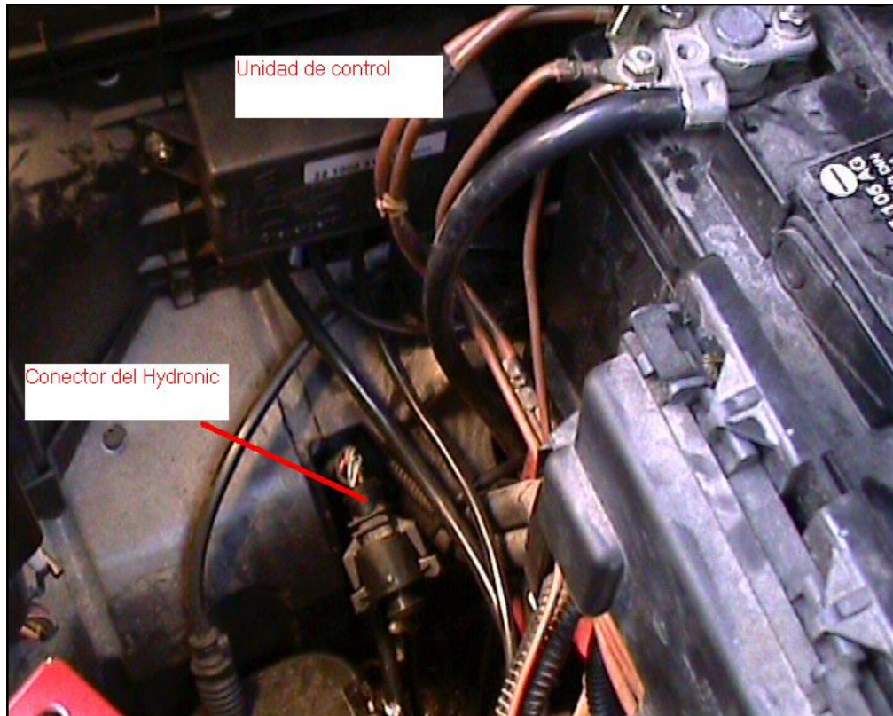
Photo 21 Unité de control, batterie et connecteur Hydronic.
