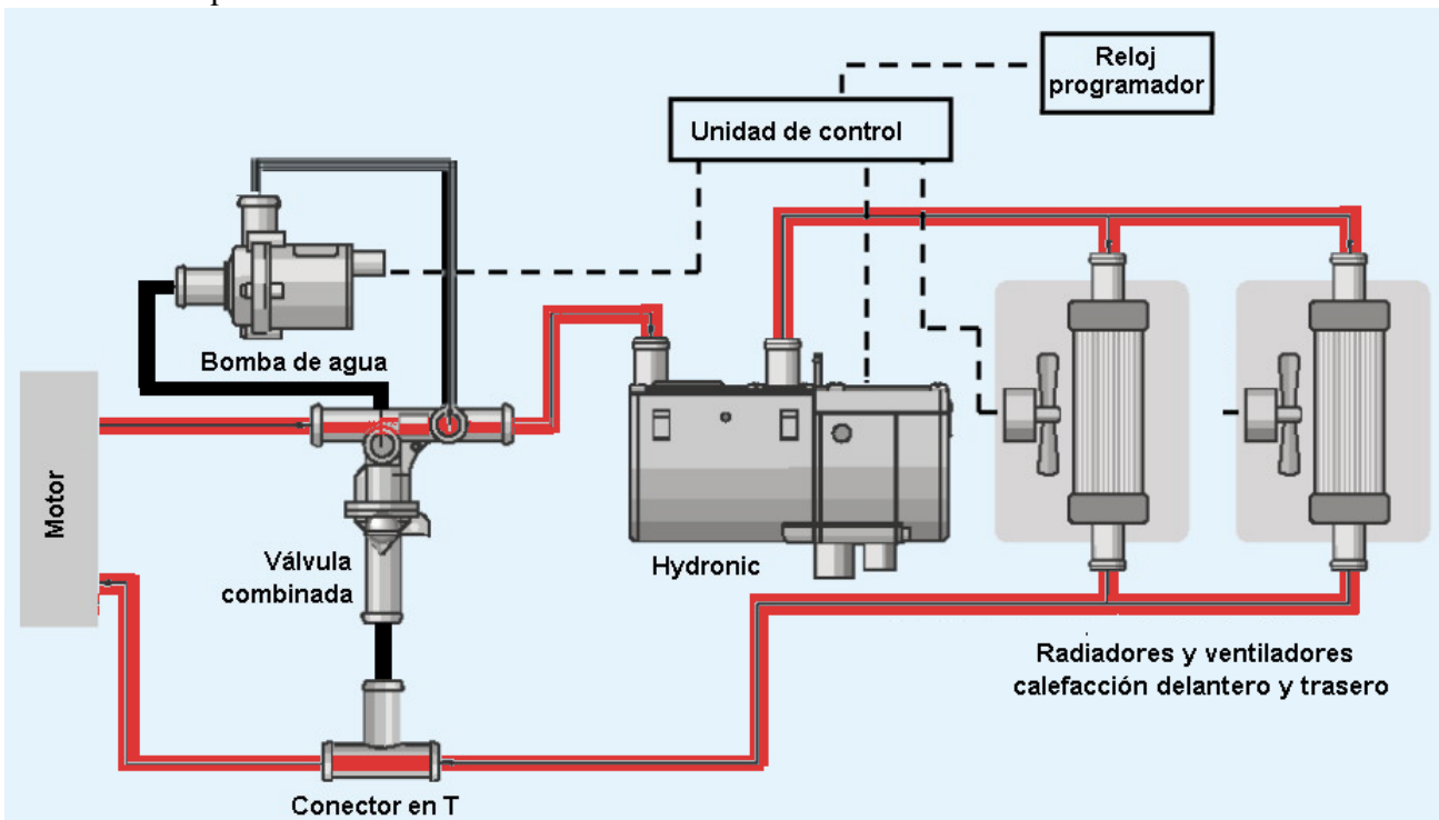
Schémas 1 : Installation du chauffage VW T4
