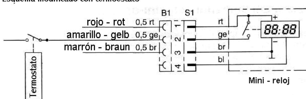
Schema 5 : Connection du thermostat
