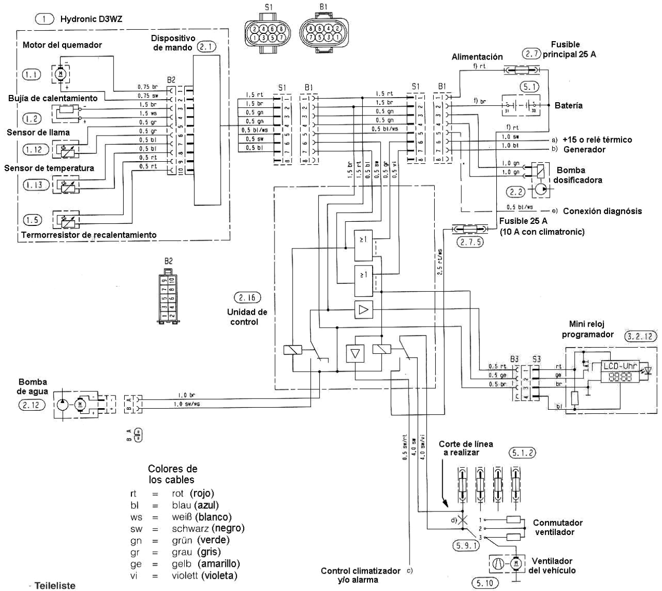
Diagrama principal de conexiones - Vehículos equipados con pre-calentador Hydronic D3WZ
