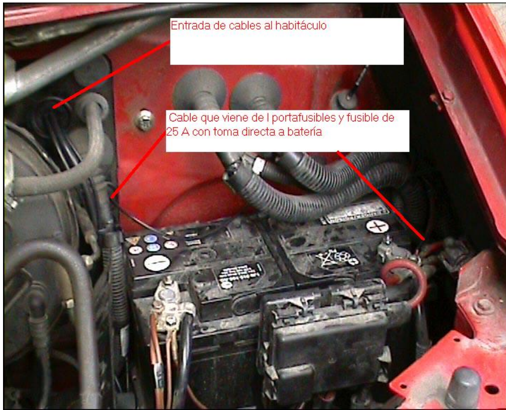
Photo 24 : Entrée des câbles dans l'habitacle.
